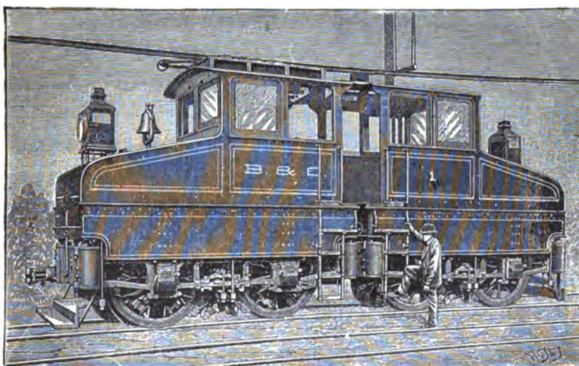
3. Электрическій локомотивъ жел. дор. Балтимора Огайо.
